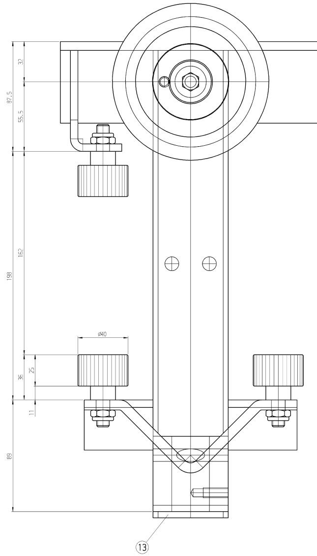
Schnitt A-A
