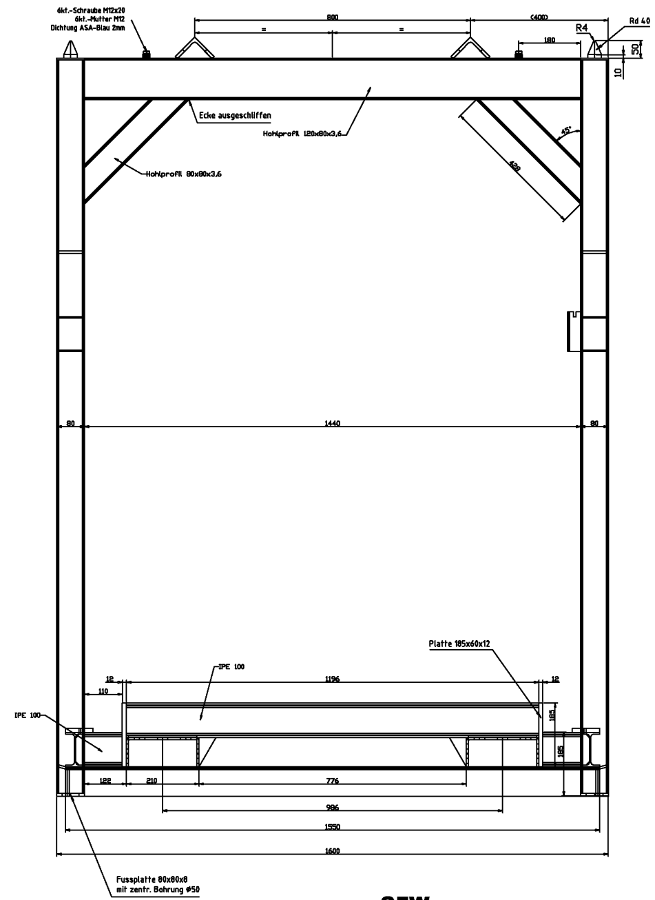
SFW Wareträger Gestell
